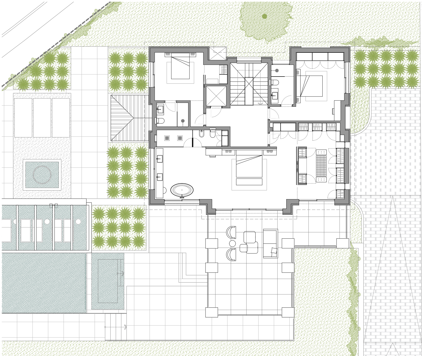
PRIMERA PLANTA / FIRST FLOOR
